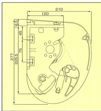
A型 壁付納まり図
