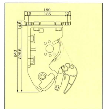
A型 ベースプレート天井付納まり図
