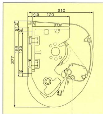
F型 ベースプレート壁付納まり図
